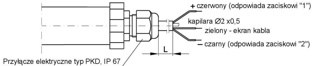
Rysunek 3. Schemat podłączenia przetwornika z przyłączem PKD.
