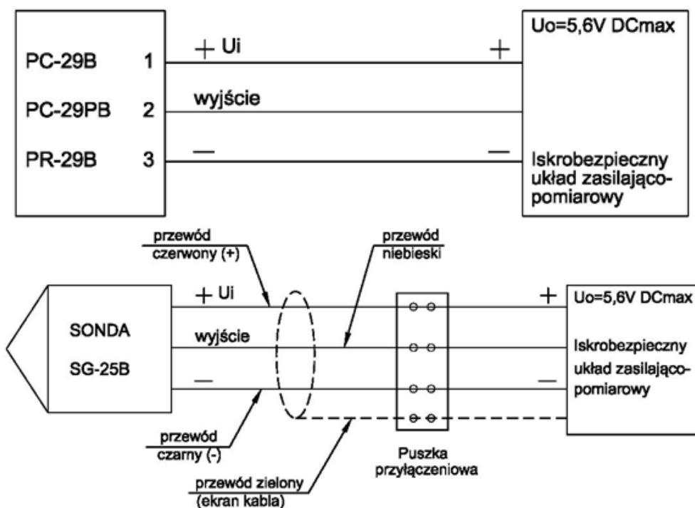
Rysunek 2. Przykłady zasilania wyrobów PC-29B, PC-29PB, PR-29B, SG-25B.
