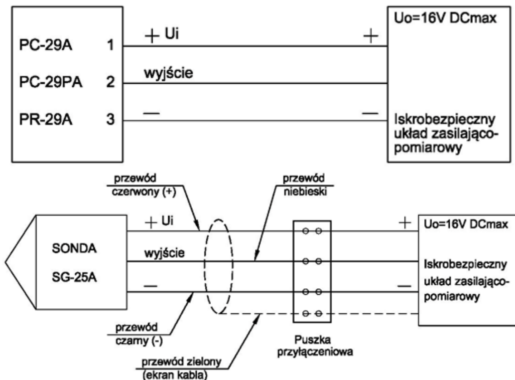
Rysunek 1. Przykłady zasilania wyrobów PC-29A, PC-29PA, PR-29A, SG-25A ze źródła o charakterystyce liniowej.
